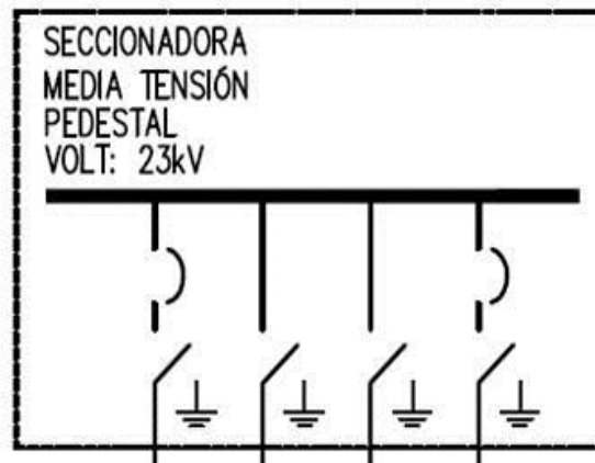
Seccionador
