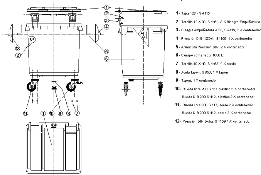
Ficha técnica del contenedor de 1,000 litros.
